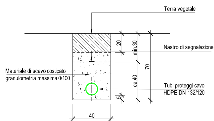
Sezione tipo profilo di scavo 1:20
