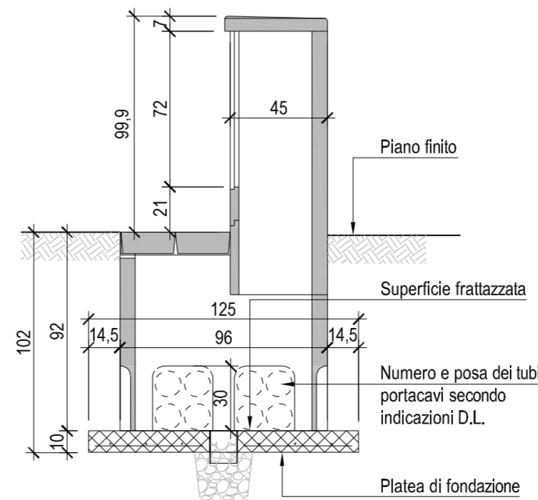
Sezione B-B 1:25
