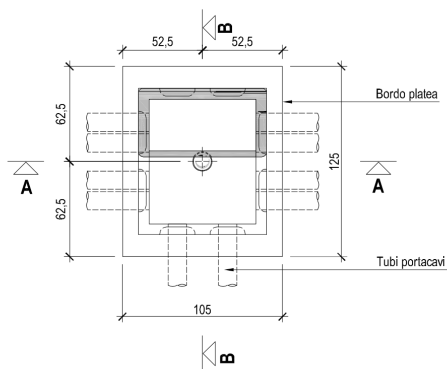
Pianta 1:25
