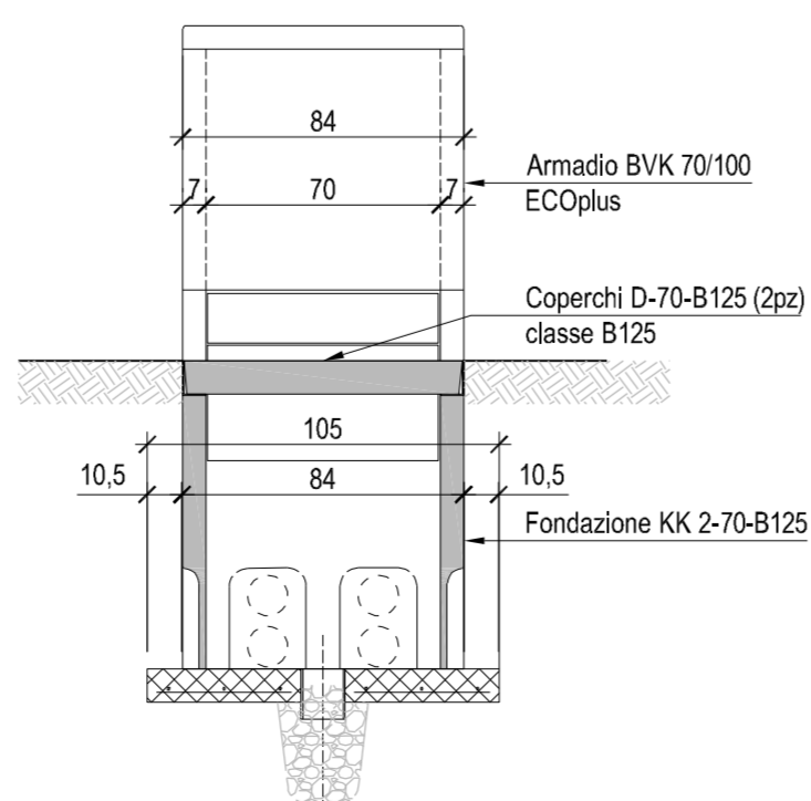
Sezione A-A 1:25
